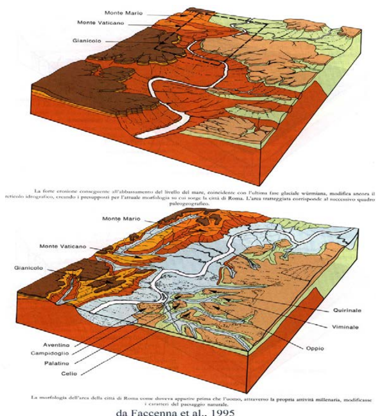
Fig. 2.2 – Evoluzione del Paleotevere
