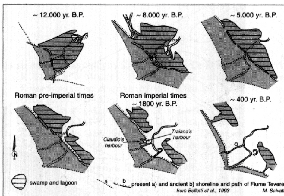
Fig. 2.3 – Evoluzione del delta del F. Tevere
